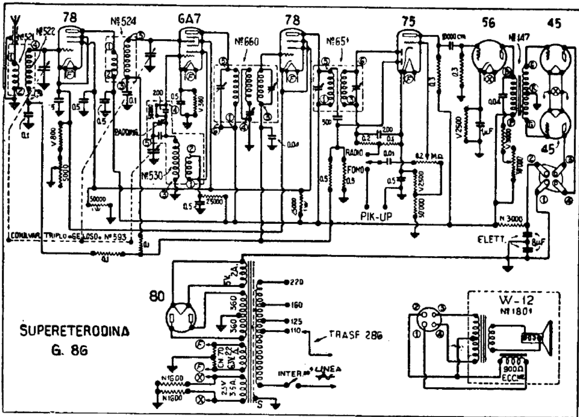
S. A. GELOSO. — Mod. G. 86. — Super monogamma con 45 finali in controfase. — Media frequenza: 348 kHz. — Produzione 1933.
